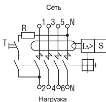
Рисунок 4 – Схема электрическая принци- пальная четырехполюсных ВД
