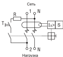
Рисунок 3 – Схема электрическая принци- пальная двухполюсных ВД
