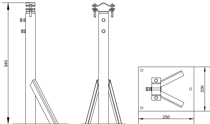
Рисунок / Figure 1 – Габаритные размеры / Overall dimensions
