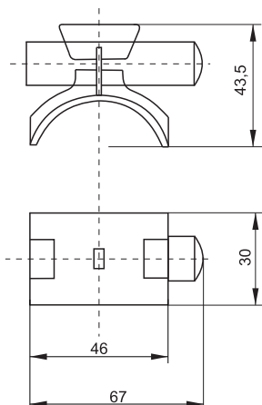
Рисунок / Figure / Сурет 1 – Габаритные и установочные размеры ДФ / Overall and installation dimensions / ҚБ-ның габариттік және орнату өлшемдері
