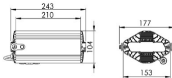
Рисунок 1 Общий вид светильника «L-lego II 30» Подвесное крепление
