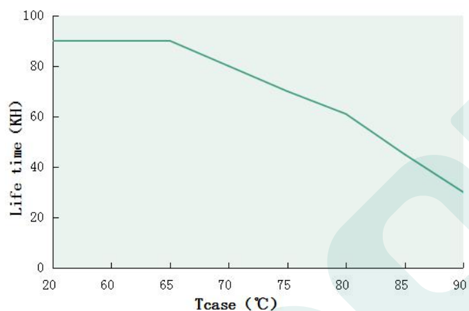
Tcase VS Lifetime(DL-240W-A/P/X-MXG)
