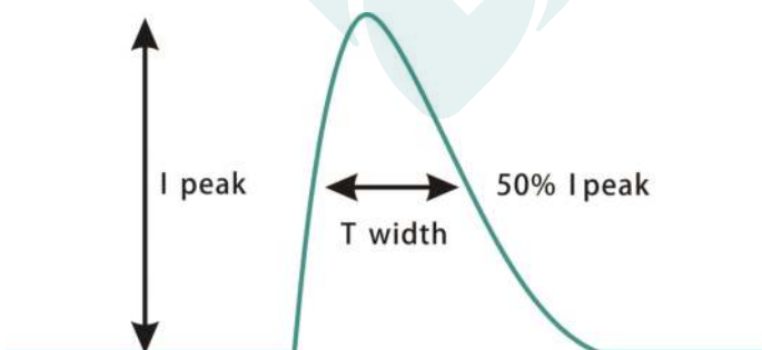
Inrush Current (DL-240W-A/P/X-MXG)
