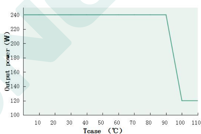
Output power VS Tcase (DL-240W-A/P/X-MXG)
