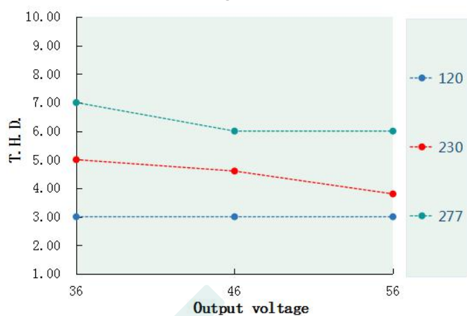
T.H.D. VS Output voltage(DL-240W-V56A/P/X-MXG)
