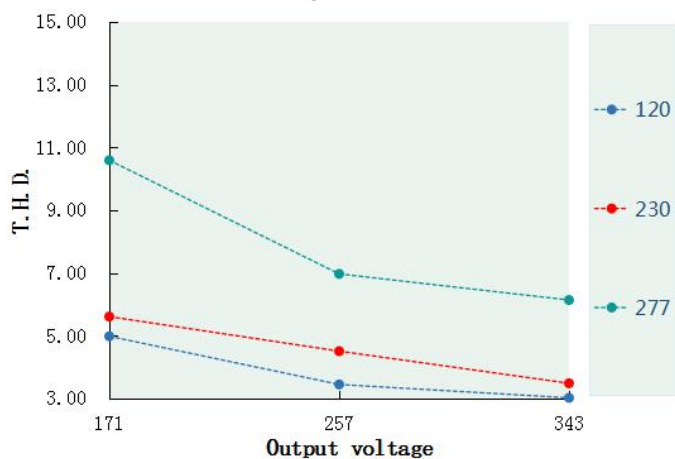
T.H.D. VS Output voltage(DL-240W-V343A/P/X-MXG)
