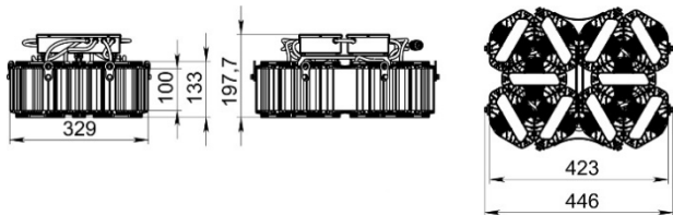
Рисунок 1 Общий вид светильника «L-lego II 500» Подвесное крепление
