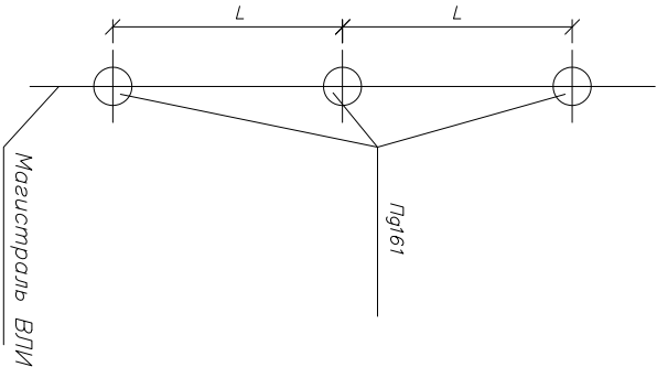
Схема установк и опор на ВЛИ
