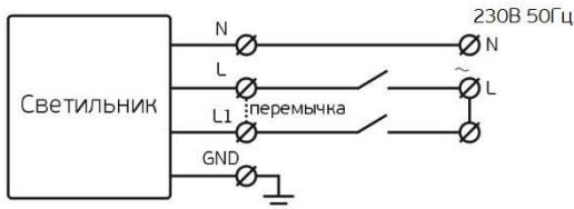
Рисунок 2 Схема подключения светильника
