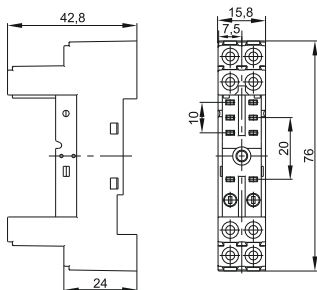
a) IMR-470-ML-2-SOC-0000-0GV
