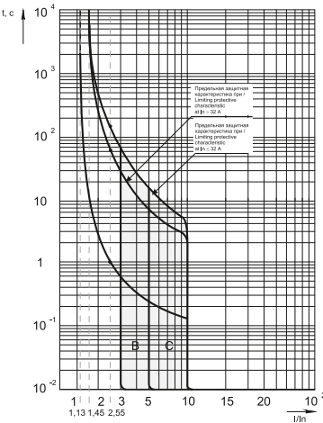
Времятоковые характеристики выключателей / Time-current characteristics of RCBO
