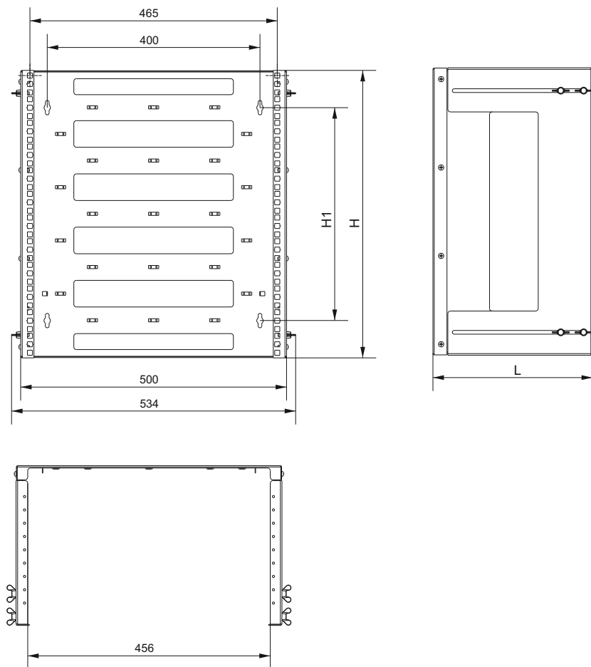
Рисунок 1 – Внешний вид рамы / Appearance of the frame / Рама сыртқы түрі
