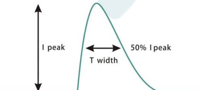
Inrush current(DL-150W-A/P/X-MXG)
