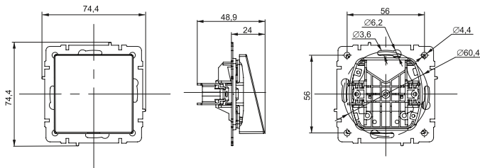
Рисунок 1 – Габаритные и установочные размеры вывода кабеля / Figure 1 – Overall and installation dimensions of the cable outlet / 1-сүрөт – Кабелды шығарудың габаритті және орнату өлшемдері / Figura 1 – Dimensiunile generale și de instalare ale ieșirii cablului / ნახატი 1 – კაბელის გამომყვანის გაბარიტული და საყენებელი ზომები / 1-сүрөт – Кабелдин чыгуусунун көлөм жана орнотулуучу өлчөмдөрү / Расми 1 – Андозаи умумӣ ва насбии даҳанаи кабел / 1-rasm – Kabel rozetkasinings gabaritlari bo'yicha va o'rnatish natijasidagi o'lchamlari
