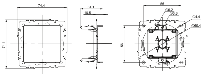
Рисунок 2 – Габаритные и установочные размеры заглушки / Figure 2 – Overall and installation dimensions of the plug / 2-сүрөт – Битеуштүң габариттү және орнату өлшемдери / Figura 2 – Dimensiunile generale și de instalare ale fișei / ნახატი 2 – სახშობის გაბარიტული და საყენებელი ზომები / 2-сүрөт – Тыгындын көлөм жана орнотулуучу өлчөмдөрү / Расми 2 – Андозаи умумий ва насбии ҷарғӯш / 2 rasm Zaglushkaning gabaritlari bo'yicha va o'rnatish natijasidagi o'lchamlari
