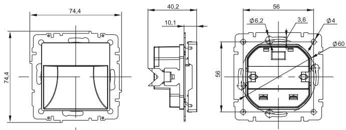
Рисунок 2 – Габаритные размеры / Figure 2 – Overall dimensions / 2-сურет – Габаритი өлшемдери / Figura 2 – Dimensiunile și dimensiunile de instalare / ნახატი 2 – გაბარიტული ზომები / 2-сურет – Көлем өлчөмдөрү / Расми 2 – Андозаи умумӣ / 2-rasm – Gabaritli va o'rnatishdagi o'lchamlari
