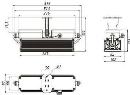
Рисунок 1 Общий вид светильника «L-industry NEW 12/Em» поворотное крепление
