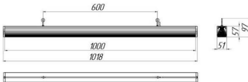
Рисунок 1 Светильник «L-fusion Office» 1,0 м
