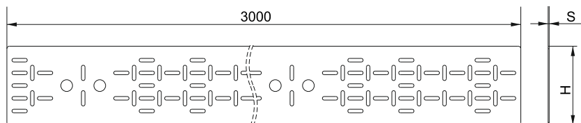
Рисунок 2 – Вставка донная для лотка LESTA 3000 / Figure 2 – Bottom ferrule for LESTA tray 3000 / 2 -keste – LESTA 3000 naağa arналğan tüptik endirmesi / Рисунок 2 – Вставка донна для лотка LESTA 3000
