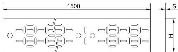
Рисунок 1 – Вставка донная для лотка LESTA 1500 / Figure 1 – Bottom ferrule for LESTA tray 1500 / 1 -keste – LESTA 1500 naağa arналğan tüptik endirmesi / Рисунок 1 – Вставка донна для лотка LESTA 1500
