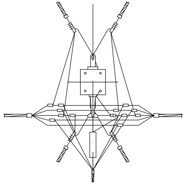
Схема отведений к входу в здания в две стороны 2х2 жилы СИП
