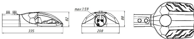
Рисунок 1 Общий вид светильника Street X1/2.0 с консольным креплением.
